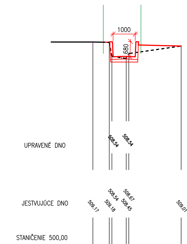
PRIEČNY REZ 22-22
