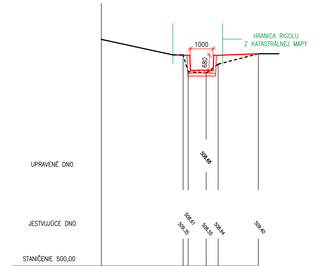
PRIEČNY REZ 21-21
