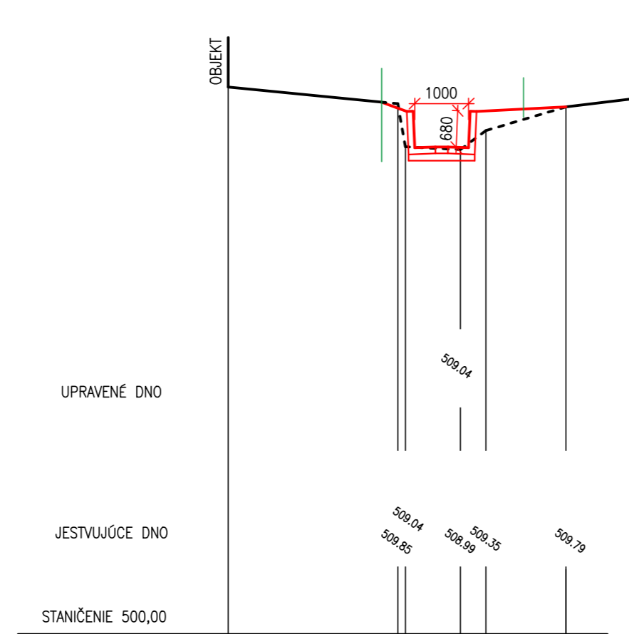
PRIEČNY REZ 19-19
