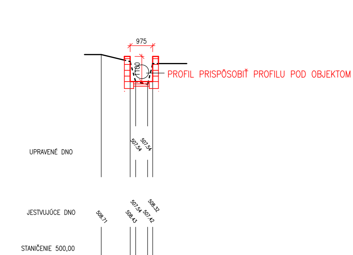
PRIEČNY REZ 24-24
