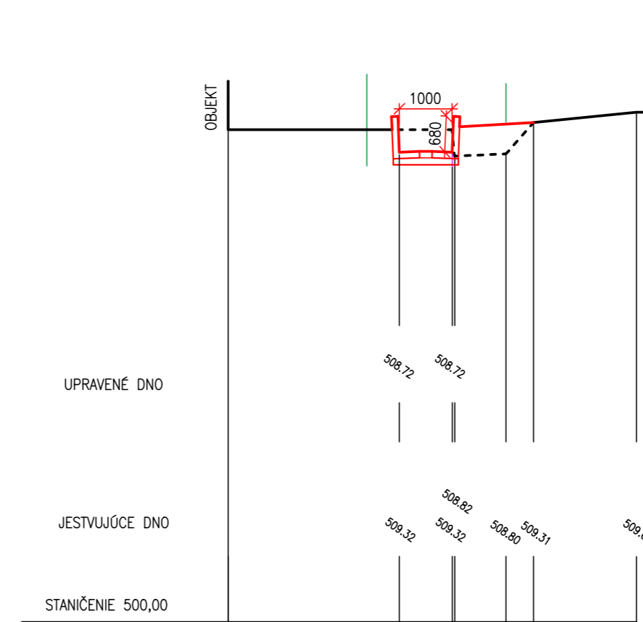
PRIEČNY REZ 20-20
