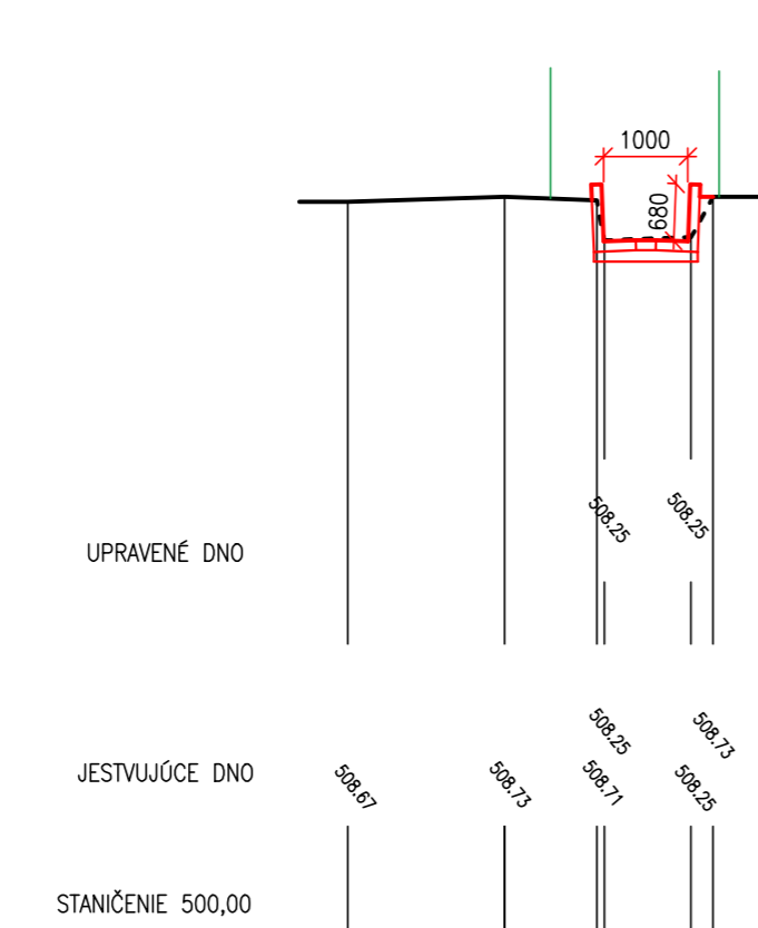
PRIEČNY REZ 23-23
