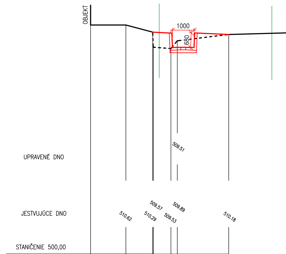
PRIEČNY REZ 18-18
