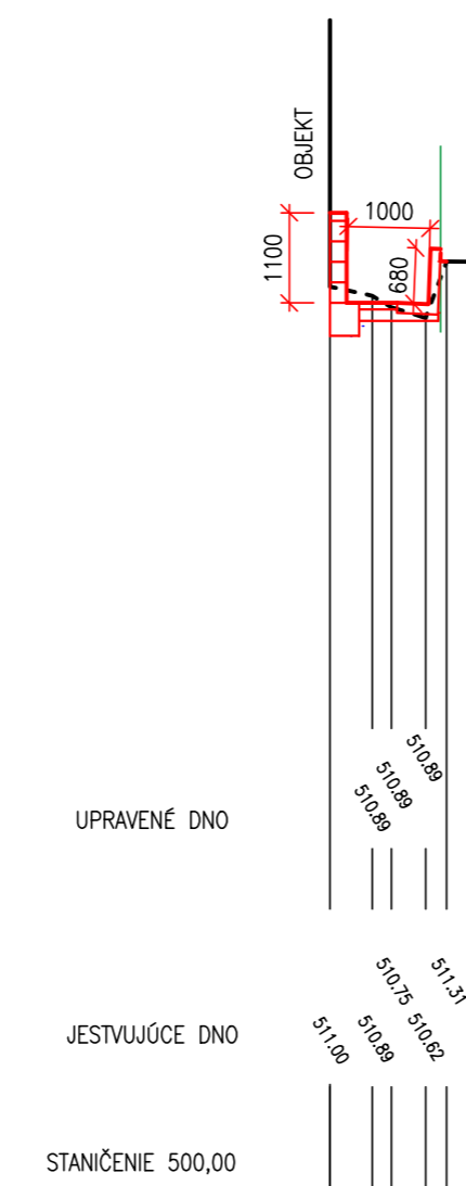
PRIEČNY REZ 11-11
